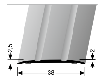
438 SK ÜBERGANGSPROFIL CONNECTING PROFILE
