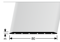
444 SK ÜBERGANGSPROFIL CONNECTING PROFILE
