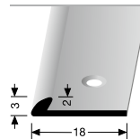
355 ABSCHLUSSPROFIL EDGE TRIM
