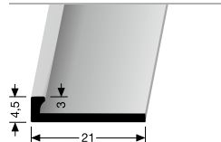
301 U ABSCHLUSSPROFIL EDGE TRIM
