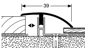
559 ANPASSUNGSPROFIL ADAPTING PROFILE
