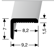
279 U WINKELPROFIL ANGLE EDGE
