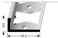
303 G DOPPEL-K PROFIL PERFORATED EDGE TRIM
