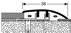
576 XL ANPASSUNGSPROFIL ADAPTING PROFILE
