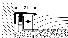
560 ABSCHLUSSPROFIL BORDER PROFILE
