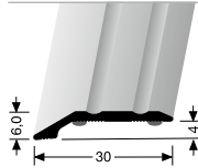
240 SK ANPASSUNGSPROFIL ADAPTING PROFILE
