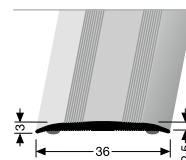
440 SK ÜBERGANGSPROFIL CONNECTING PROFILE
