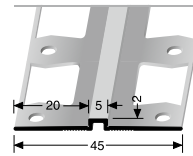
170 G VERBINDER CONNECTOR
