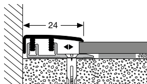
577 XL ABSCHLUSSPROFIL BORDER PROFILE
