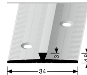
365 ABSCHLUSSPROFIL EDGE TRIM
