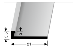
299 U ABSCHLUSSPROFIL EDGE TRIM
