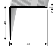
229 U WINKELPROFIL ANGLE EDGE
