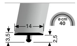
289 U T-PROFIL T-PROFILES
