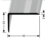
228 SK WINKELPROFIL ANGLE EDGE
