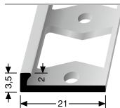
299 G DOPPEL-K PROFIL PERFORATED EDGE TRIM
