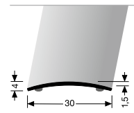
459 SK ÜBERGANGSPROFIL CONNECTING PROFILE
