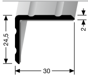
234 SK WINKELPROFIL ANGLE EDGE
