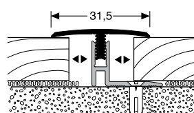
561 ÜBERGANGSPROFIL CONNECTING PROFILE
