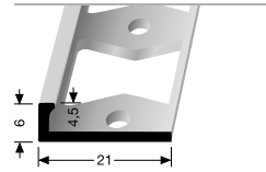
302 G DOPPEL-K PROFIL PERFORATED EDGE TRIM
