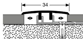
578 XL ÜBERGANGSPROFIL CONNECTING PROFILE
