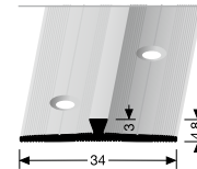
365 EINFASSPROFIL EDGE TRIM
