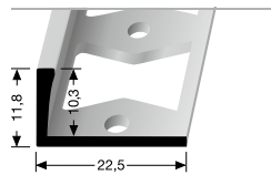
304 G DOPPEL-K PROFIL PERFORATED EDGE TRIM
