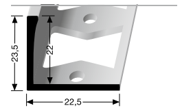
309 G DOPPEL-K PROFIL PERFORATED EDGE TRIM
