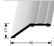
241 SK ANPASSUNGSPROFIL ADAPTING PROFILE
