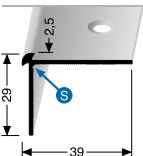
870 TREPPENKANTENPROFIL STAIR NOSING
