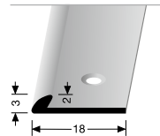
355 ABSCHLUSSPROFIL BORDER PROFILE
