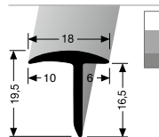
294 EINFASSPROFIL EDGE TRIM
