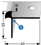
875 TREPPENKANTENPROFIL STAIR NOSING
