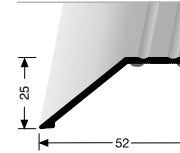
245 SK ANPASSUNGSPROFIL ADAPTING PROFILE
