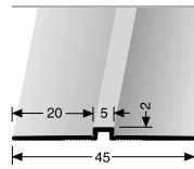
170 U VERBINDER CONNECTOR
