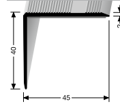
229 SK WINKELPROFIL ANGLE EDGE
