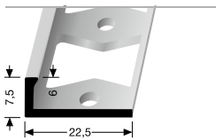
307 G DOPPEL-K PROFIL PERFORATED EDGE TRIM
