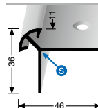
876 TREPPENKANTENPROFIL STAIR NOSING
