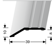
244 SK ANPASSUNGSPROFIL ADAPTING PROFILE
