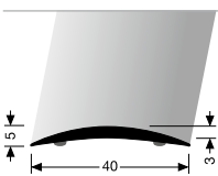
462 SK ÜBERGANGSPROFIL CONNECTING PROFILE
