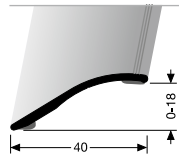
248 SK ANPASSUNGSPROFIL ADAPTING PROFILE
