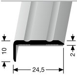
236 SK WINKELPROFIL ANGLE EDGE
