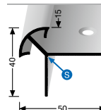
879 TREPPENKANTENPROFIL STAIR NOSING
