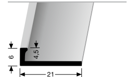
302 U ABSCHLUSSPROFIL EDGE TRIM
