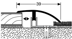
556 ANPASSUNGSPROFIL ADAPTING PROFILE
