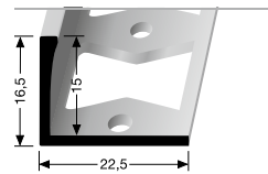
306 G DOPPEL-K PROFIL PERFORATED EDGE TRIM
