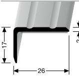
237 SK WINKELPROFIL ANGLE EDGE
