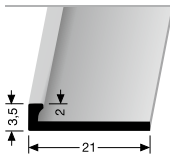
299 U ABSCHLUSSPROFIL EDGE TRIM
