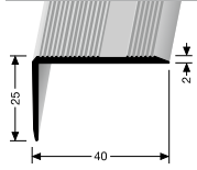
228 U WINKELPROFIL ANGLE EDGE
