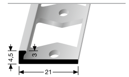
301 G DOPPEL-K PROFIL PERFORATED EDGE TRIM
